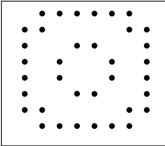
Ubicaciones LED in 42W fixture
